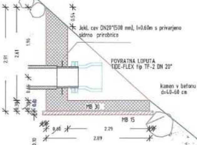
PREREZ A-A M 1:50
